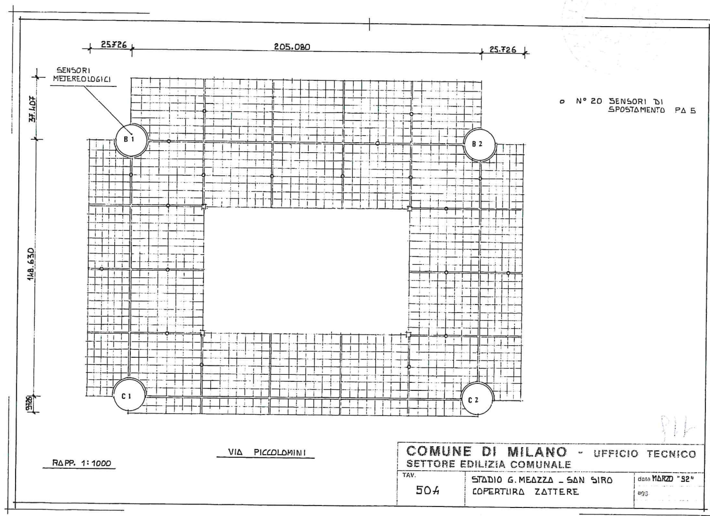
Fig. 11: La copertura
