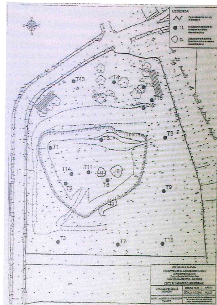
Fig.03: Indagine ambientale area cantiere M5 - Ubicazione delle trincee esplorative
