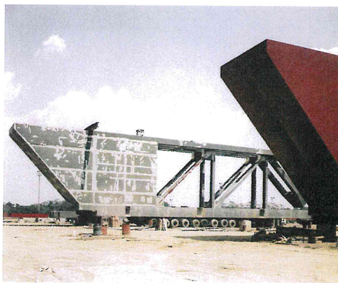
Fig. 12: Cantiere, fasi di montaggio terzo anello e copertura
