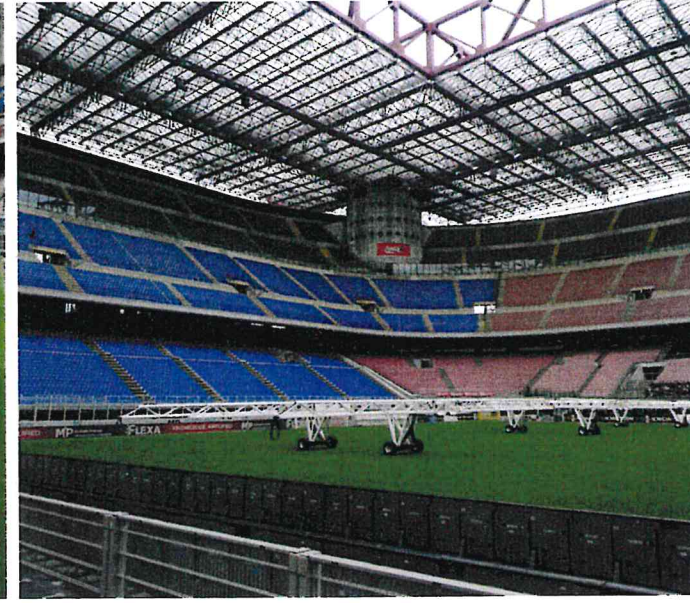
Fig. 22: La curva sud e la torre angolare di sostegno alla copertura
