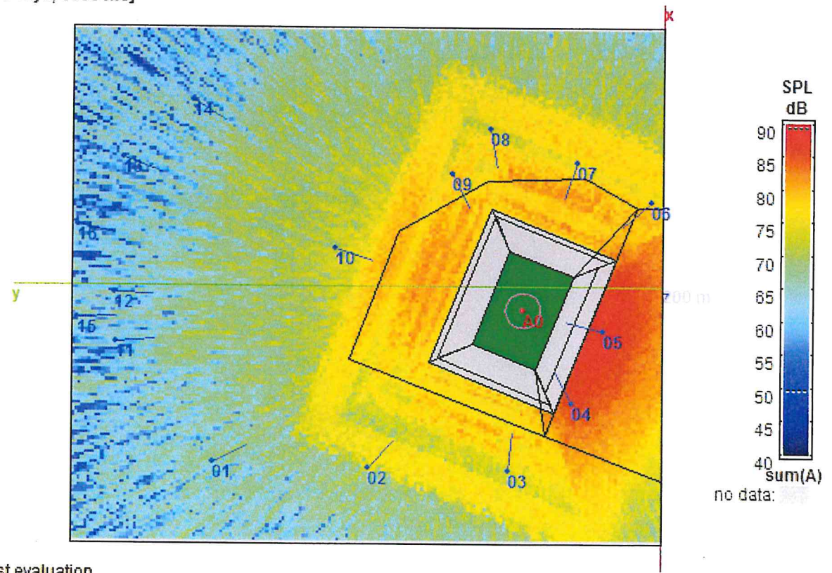
Fig. 13: Distribuzione dei livelli sonori calcolata per l'evento concerto.
