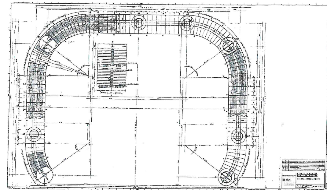
Fig. 09: Pianta tracciamento
